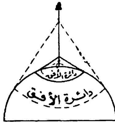
استدارة الأفق واتساعه بالارتفاع
